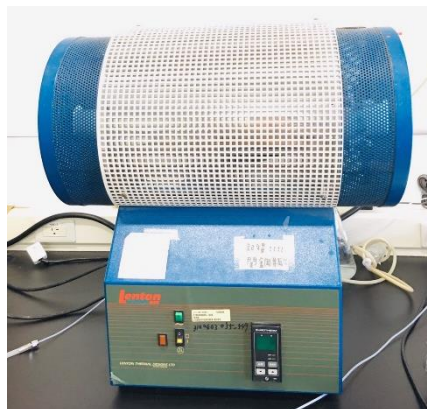
高溫爐
