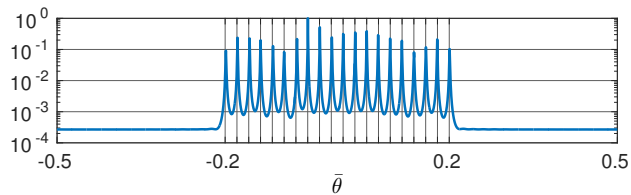
(d) Second-order super nested, D = 20 , E = 0.00082022 .
