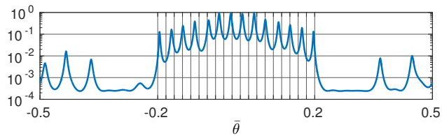
(c) Coprime array, D = 20 , E = 0.12749 .
