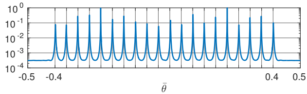
(d) Second-order super nested, D = 20 , E = 0.0010173 .
