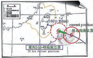
海上颱風警報發布標準示意圖 (圖片來源：中央氣象局)
