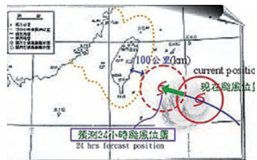
海上陸上颱風警報發布標準示意圖 (圖片來源：中央氣象局)
